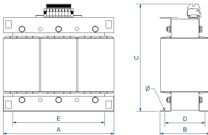
Dimensions (AxBxCxDxE): 240x145x253x125x200 mm 9
