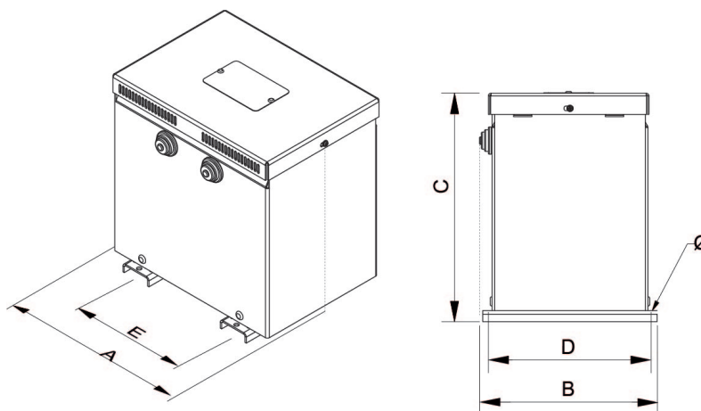
Dimensions (AxBxCxDxE): 315x230x315x205x200 mm 6Ø
