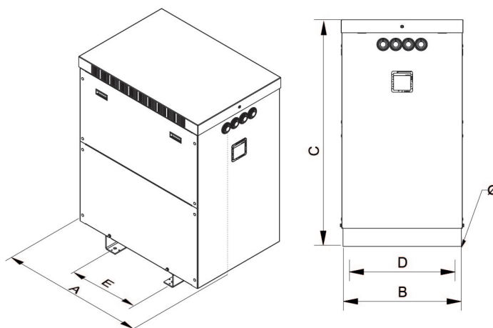
Dimensions (AxBxCxDxE): 310x230x308x205x197 mm 6Ø
