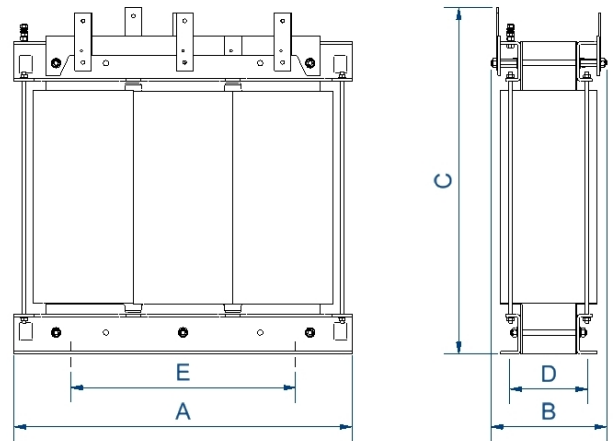
Dimensiones (AxBxCxDxE): 1020x550x880x460x470 mm 13Ø
