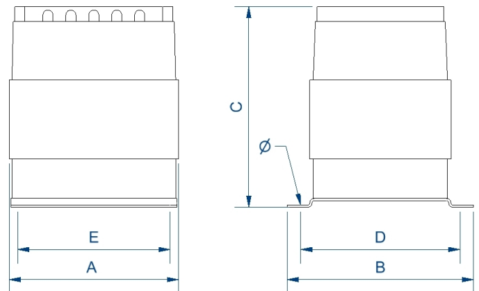
Dimensiones (AxBxCxDxE): 150x165x180x145x125 mm 7Ø
