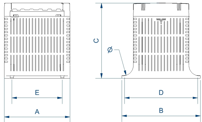
Dimensions (AxBxCxDxE): 136x162x156x146x104 mm 6∅
