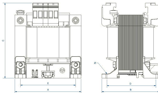
Dimensiones (AxBxCxDxE): 75x82x89,5x71x62,5 mm 6
