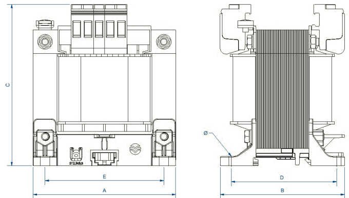
Dimensiones (AxBxCxDxE): 75x67x89,5x56x62,5 mm 6
