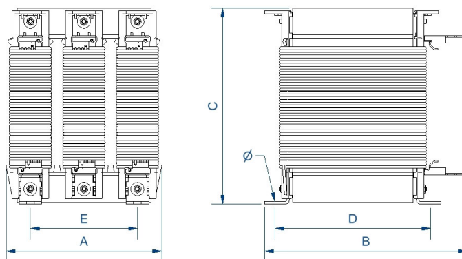
Dimensiones (AxBxCxDxE): 120x84x107x54x100 mm 6
