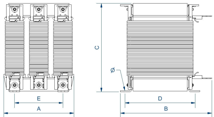
Dimensiones (AxBxCxDxE): 180x205x220,25x144x120 mm 6Ø
