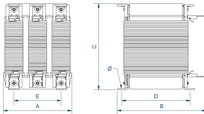
Dimensiones (AxBxCxDxE): 180x155x220,25x94x120 mm 6Ø
