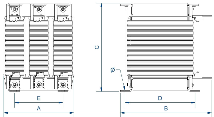
Dimensions (AxBxCxDxE): 150x155x185x94x100 mm 6Ø
