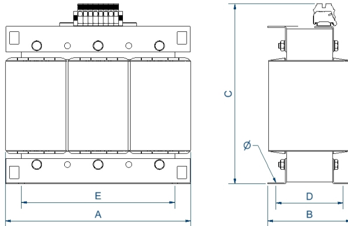
Dimensions (AxBxCxDxE): 180x94x203x76x150 mm 6∅
