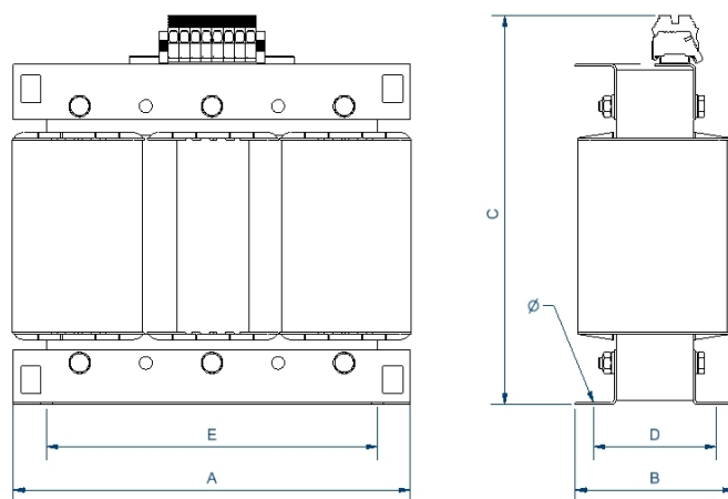
Dimensions (AxBxCxDxE): 330x154x303x145x250 mm 9Ø
