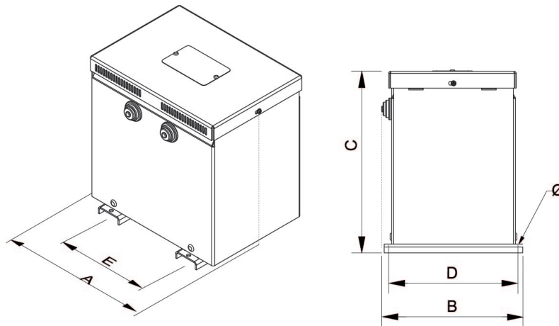
Dimensions (AxBxCxDxE): 310x230x308x205x197 mm 6Ø
