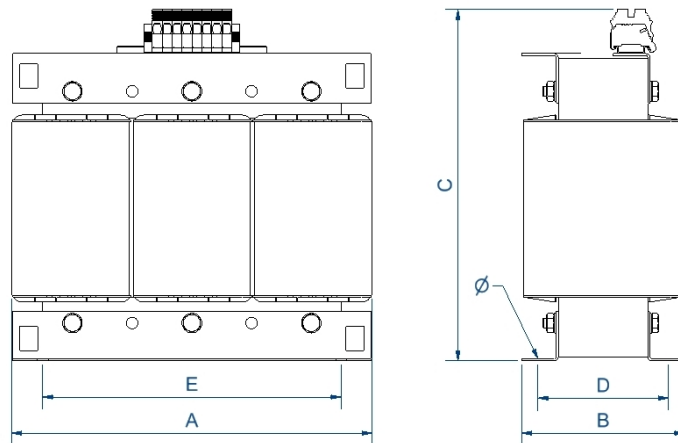
Dimensions (AxBxCxDxE): 240x143x268x125x200 mm 9Ø
